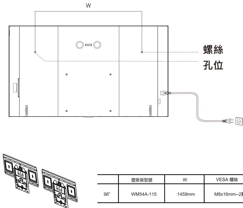
壁掛架示意圖 (需另外購買)
