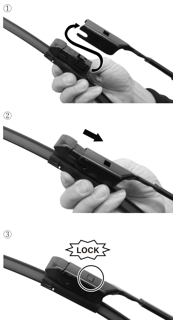
如何安裝PIAA雨刷 How to install PIAA Wiper
