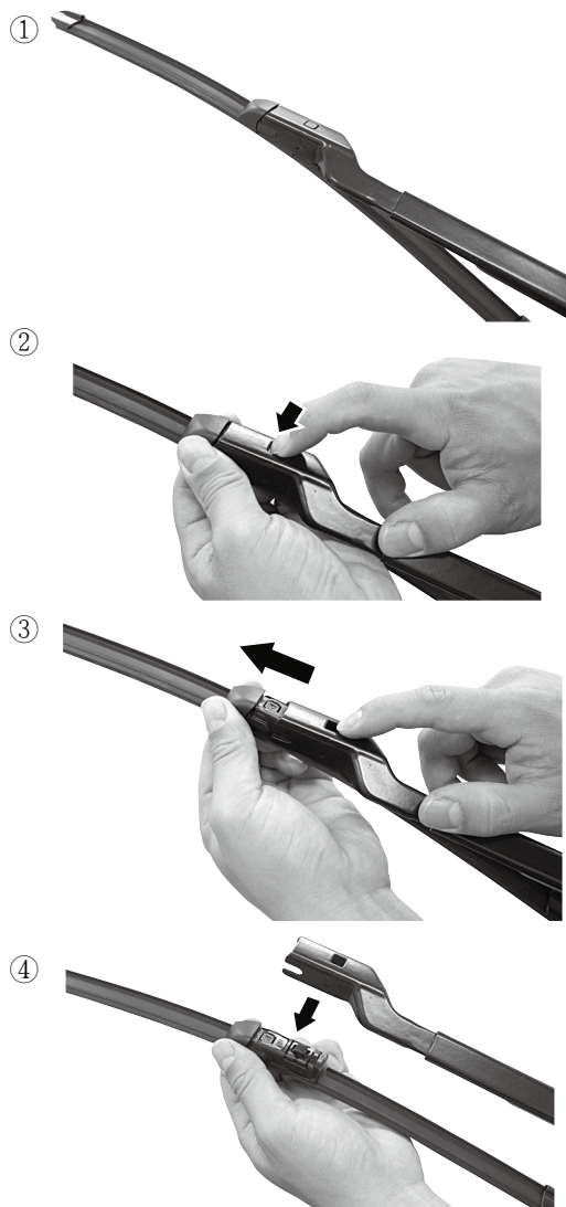
如何移除舊雨刷 How to remove old wipe
